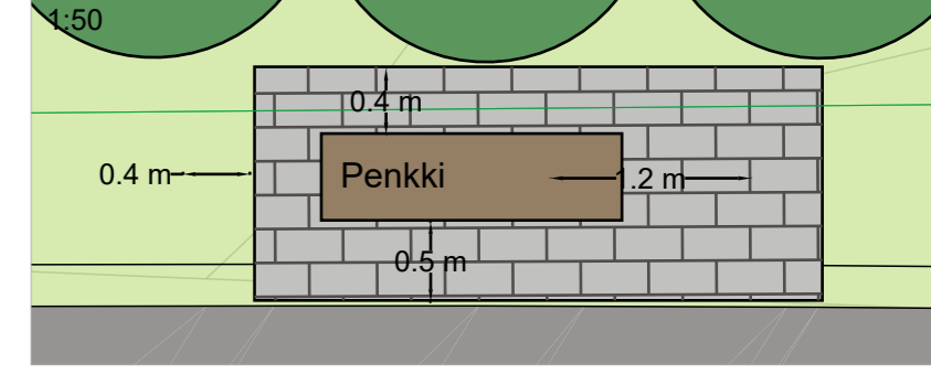
DETALJI 2: Kiveyksen mitoitus penkeille, kivimateriaali ks. työselustus
