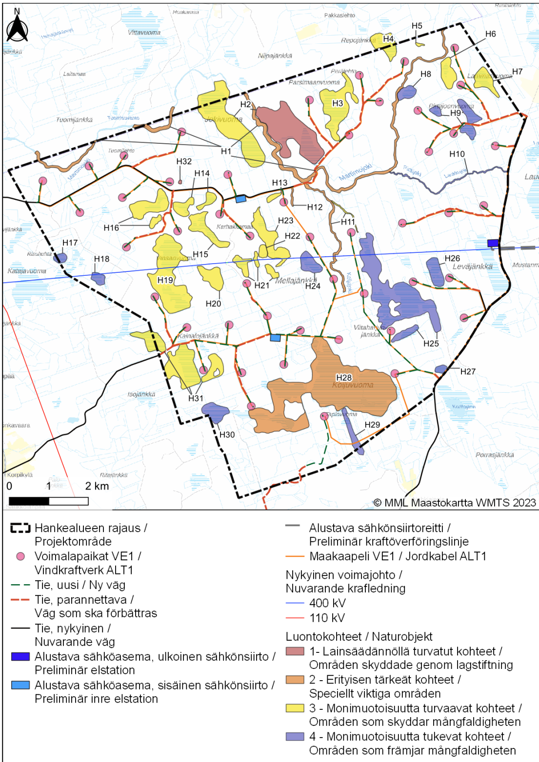
Kuva 38. Hankealueen numeroidut luontokohteet sekä voimalapaikat ja tiestö.
