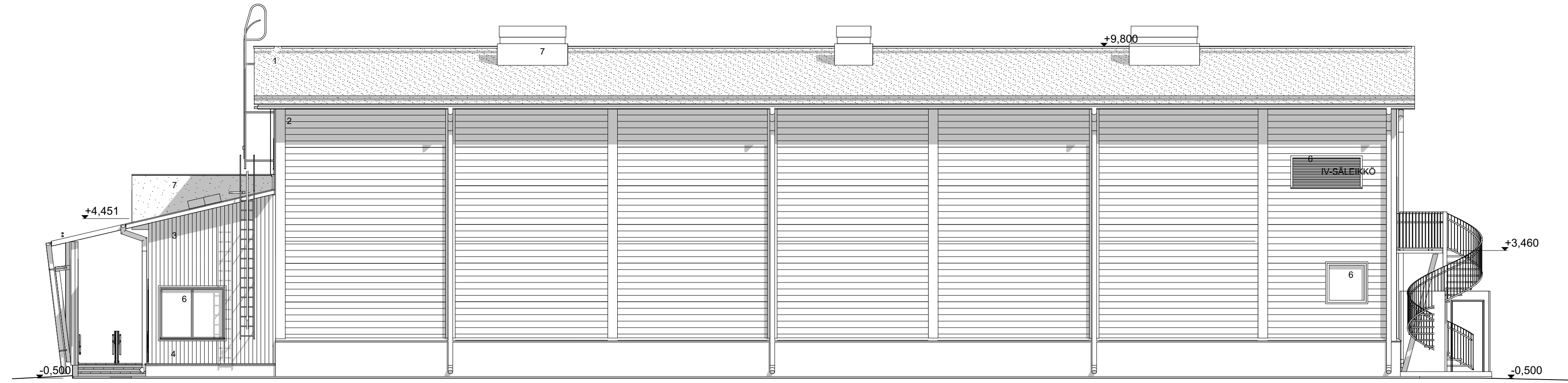
JULKISIVU ITÄÄN
