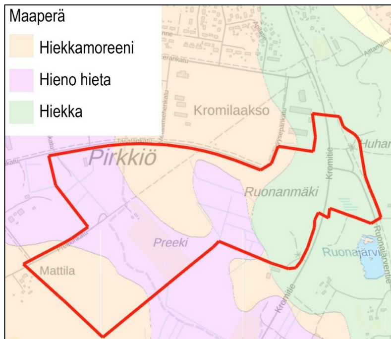
Kuva 3. Maaperä. (GTK, Maanmittauslaitos)
