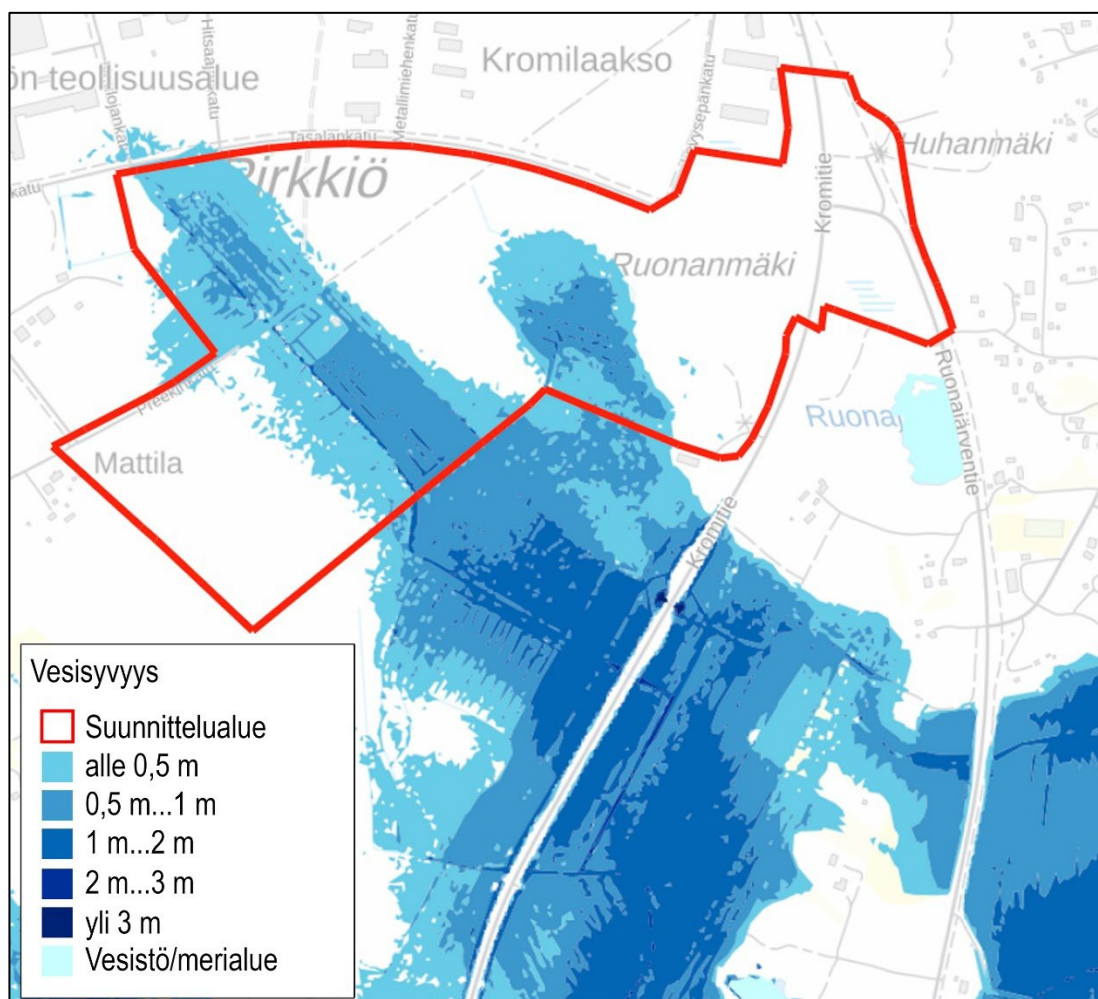
Kuva 6. Harvinaisen meritulvan (1/250a, 1 %) esiintymisalue suunnittelualueella.
