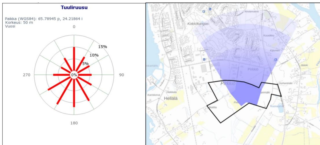
Kuva 14. Tuuliolosuhteet Kromilaaksossa osoittaa vallitsevat tuulensuunnat (etelä-lounas) ja ilmaan joutuvien mahdollisten päästöjen todennäköinen leviämismuoto alueella.
