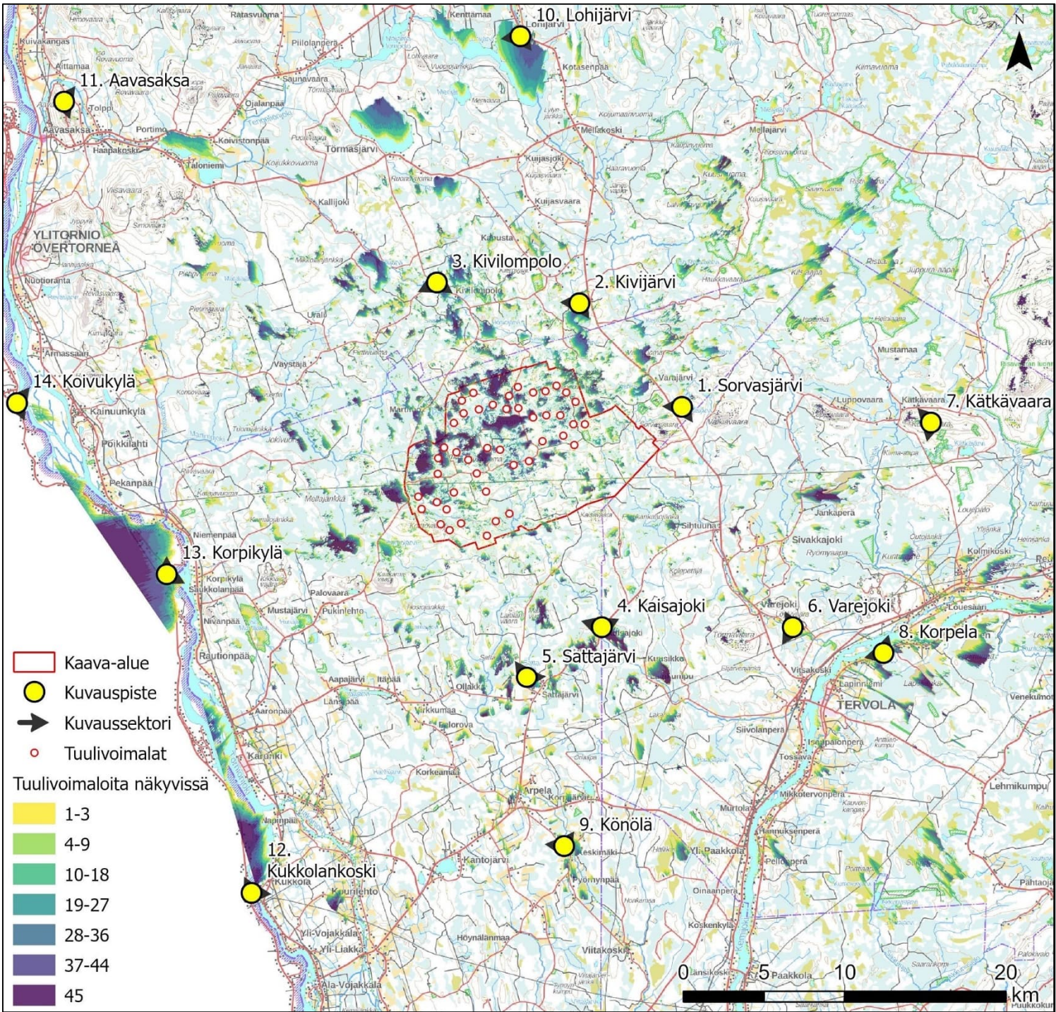
Kuvassa on esitetty havainnekuvauspisteet, kuvaussuunta kuvaussektorina sekä näkymäalueanalyysi.
