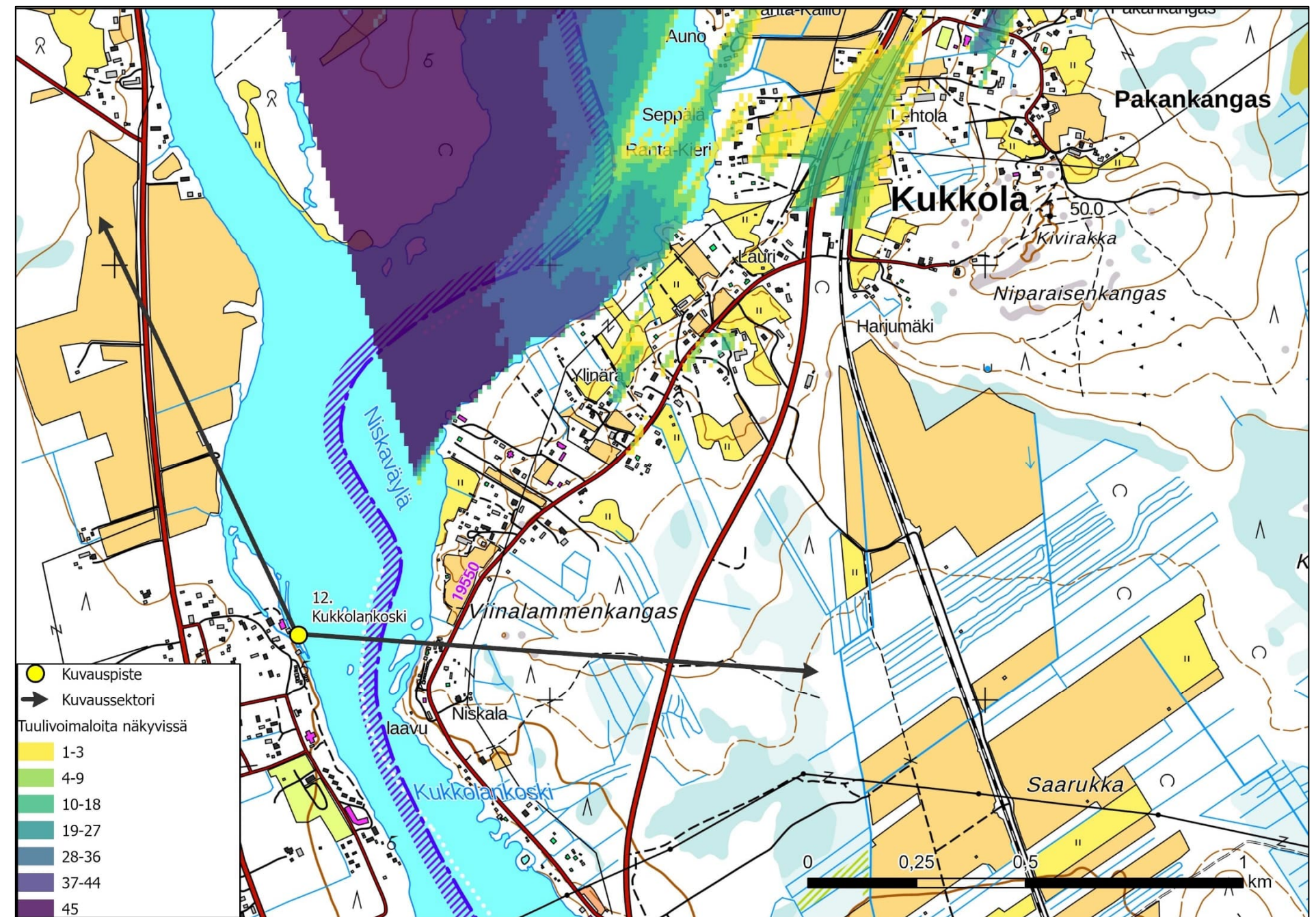
Kuva 11.1. Kukkolankosken kuvauspiste. Leikekartalla on esitetty kuvaussuunta sektorinuolilla sekä näkymäalueanalyysin mukaan näkyvien voimaloiden määrä kuvauspisteelle.
