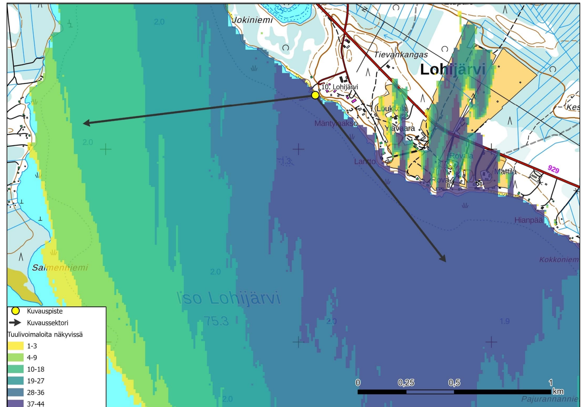
Kuva 10.1. Lohijärven kuvauspiste. Leikeydellä on esitetty kuvaussuunta sektorinuoilla sekä näkymäalueanalyysin mukaan näkyvien voimaloiden määrä kuvauspisteelle.
