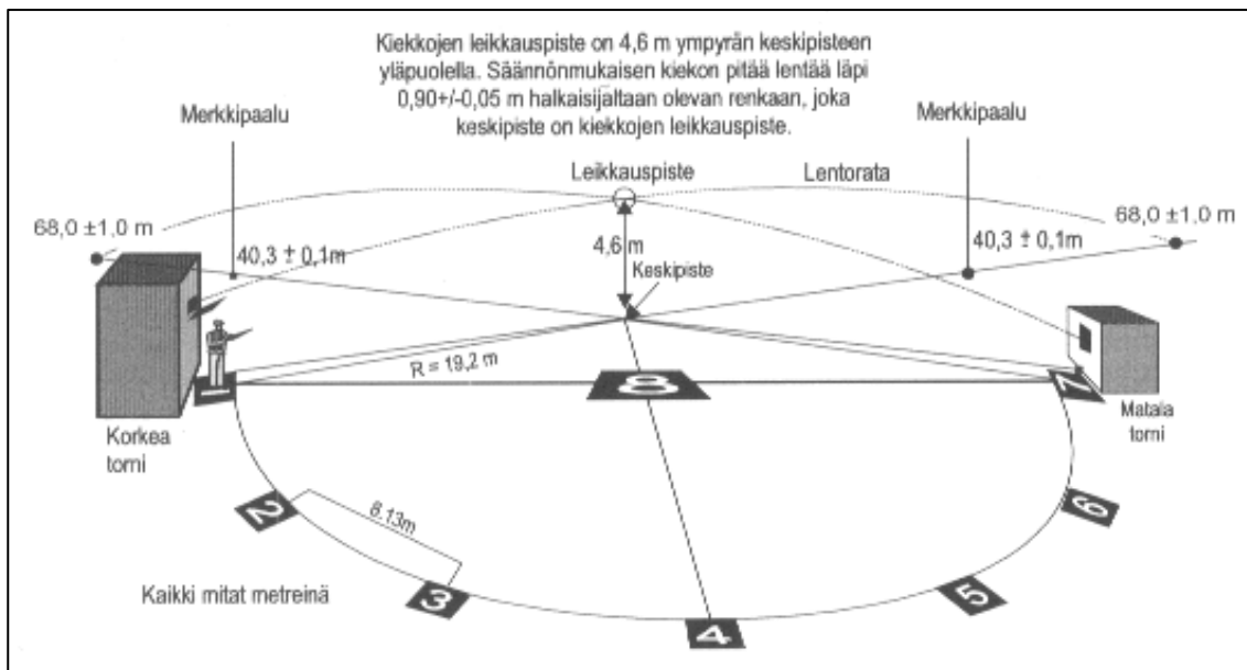
Kuva 17. Skeet-radan periaatepiirros. (Suomen ampumaurheiluliitto 2005)
