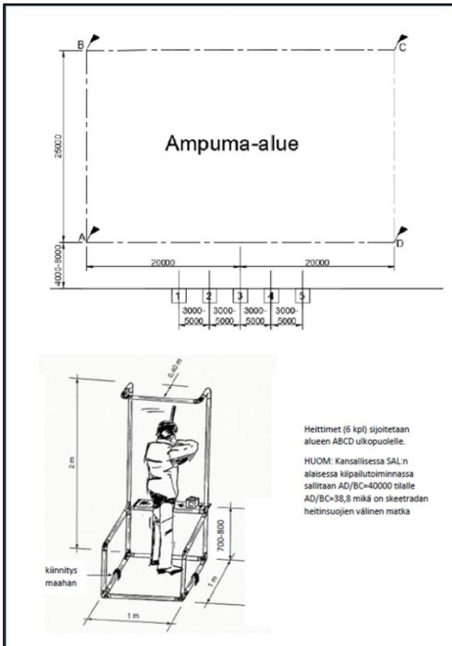
Kuva 19. Kuva Compak-sporting-radan ja yksittäisen ampumapaikan sääntöjen mukaisesta mitoitus- Hietakaulan radalla ampuma-alue rajataan sääntöjen mukaista pienemmäksi.
