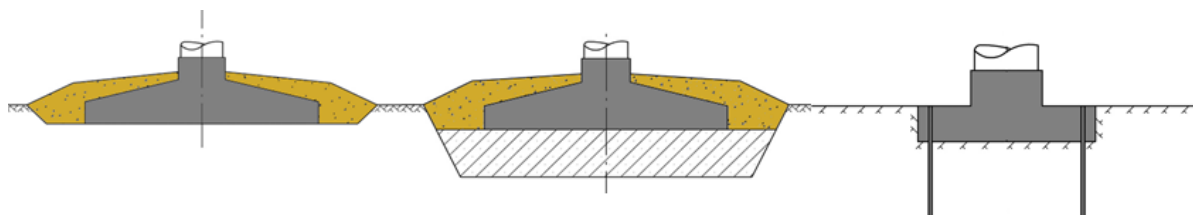
Kuva 15. Tuulivoimalat voidaan perustaa useilla eri tavoilla. Periaatekuvat maanvaraisesta teräsbetoniperustuksesta, teräsbetoniperustuksesta massanvaihdoilla sekä kallioankkuroidusta teräsbetoniperustuksesta.
