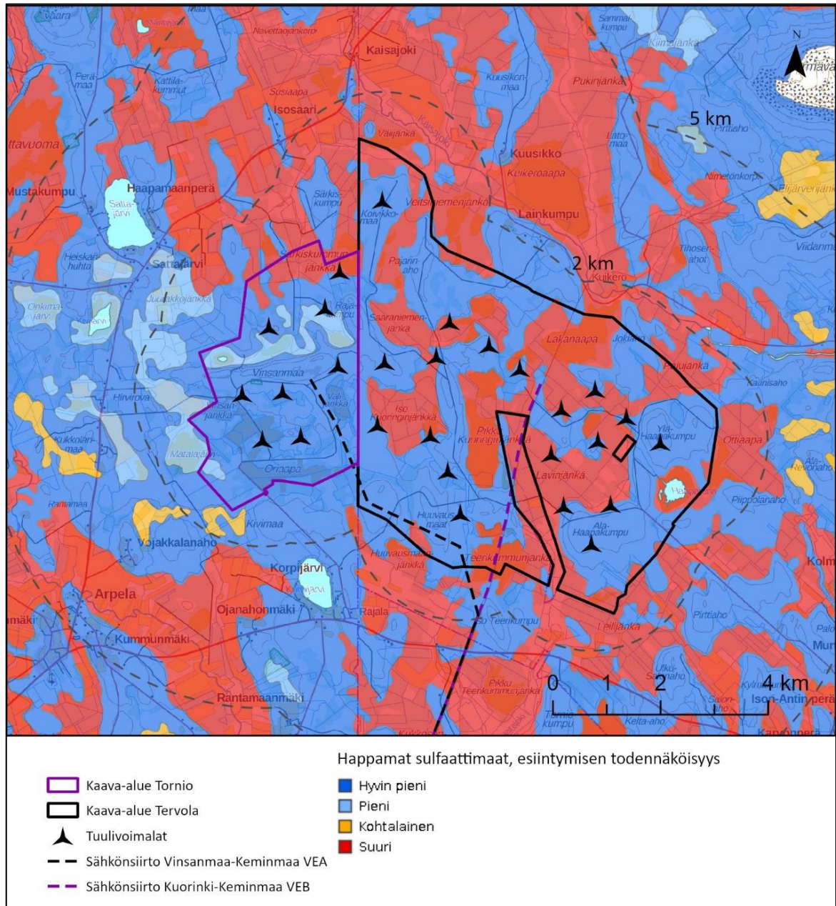
Kuva 4.15. Happamat sulfaattimaat suunnittelualueella ja sen läheisyydessä.
