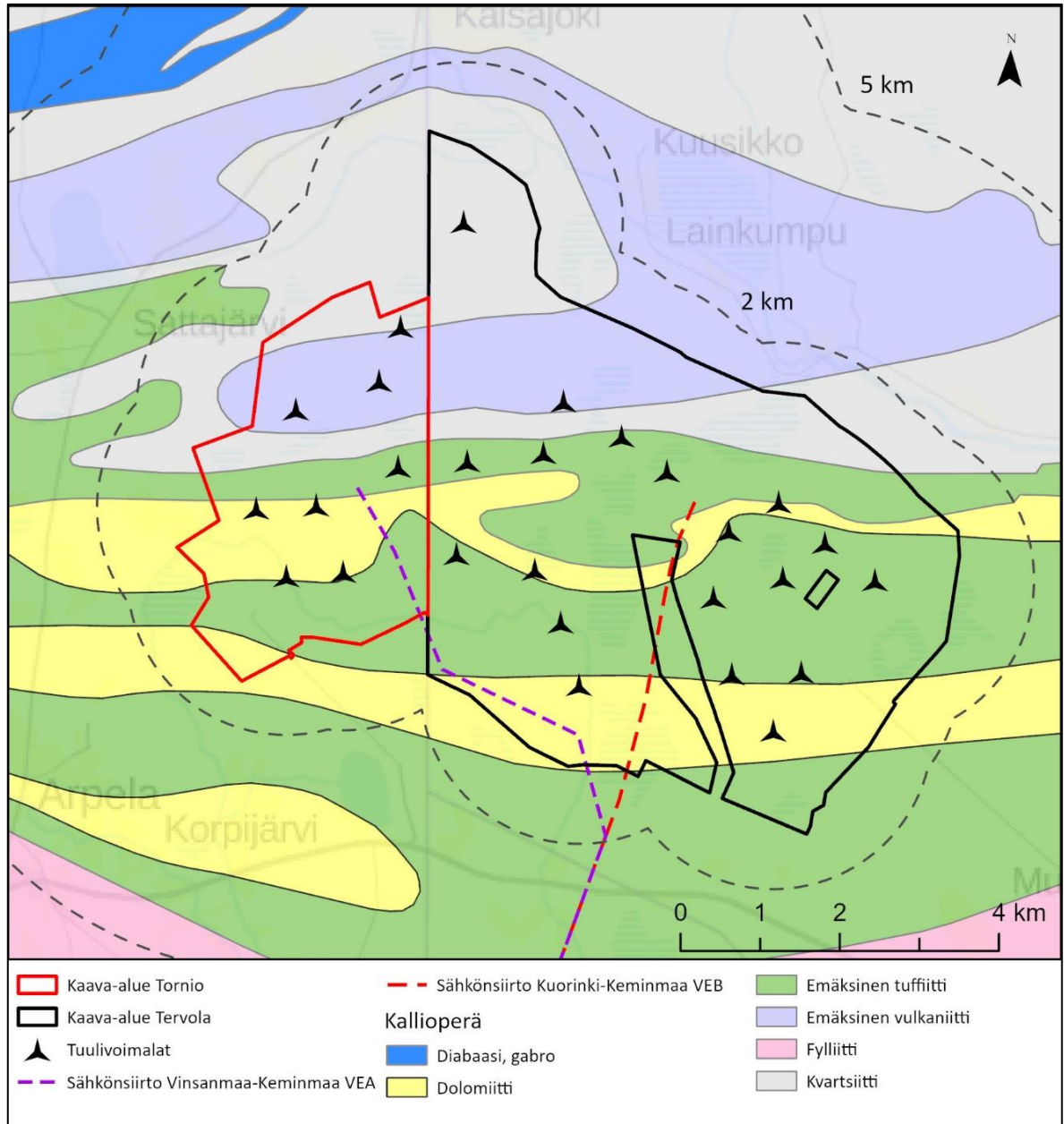
Kuva 4.13. Kallioperä suunnittelualueella ja sen ympäristössä (GTK).
