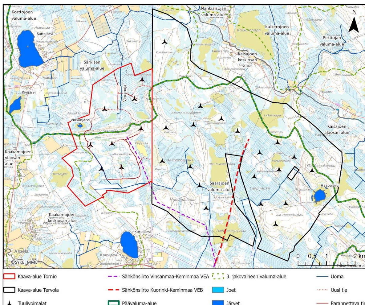
Kuva 4.18. Suunnittelualueen sijoittuminen 3. jakovaiheen valuma-alueille ja pintavesialueet (Syke).
