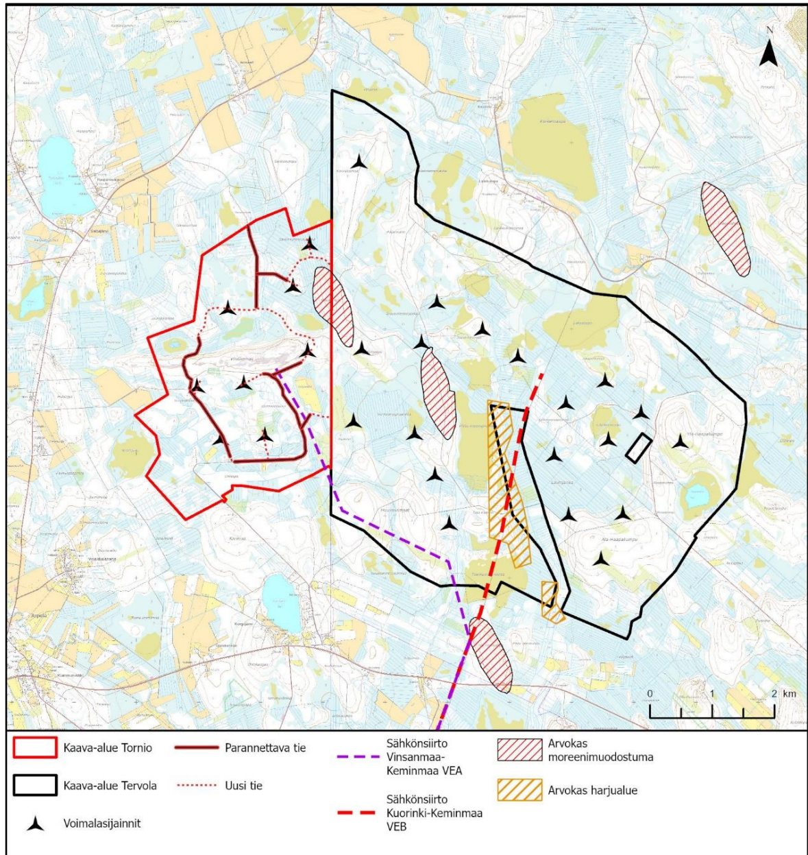
Kuva 4.16. Alueella esiintyvät arvokkaat geologiset kohteet.
