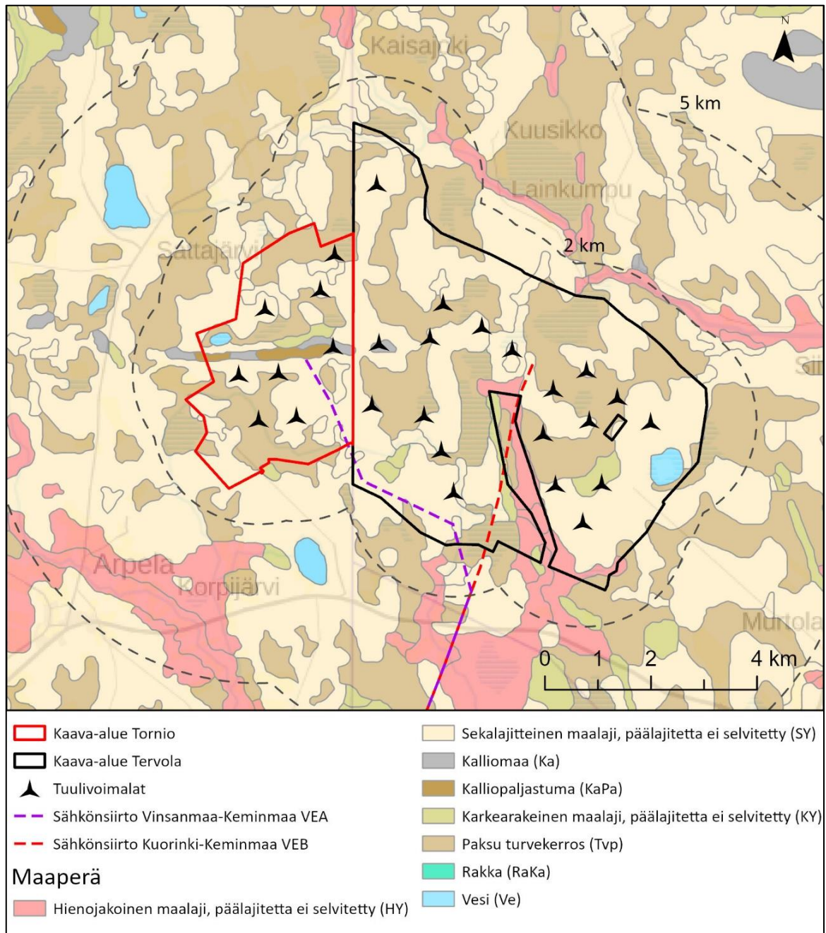
Kuva 4.14. Maaperä suunnittelualueella ja sen ympäristössä (GTK).
