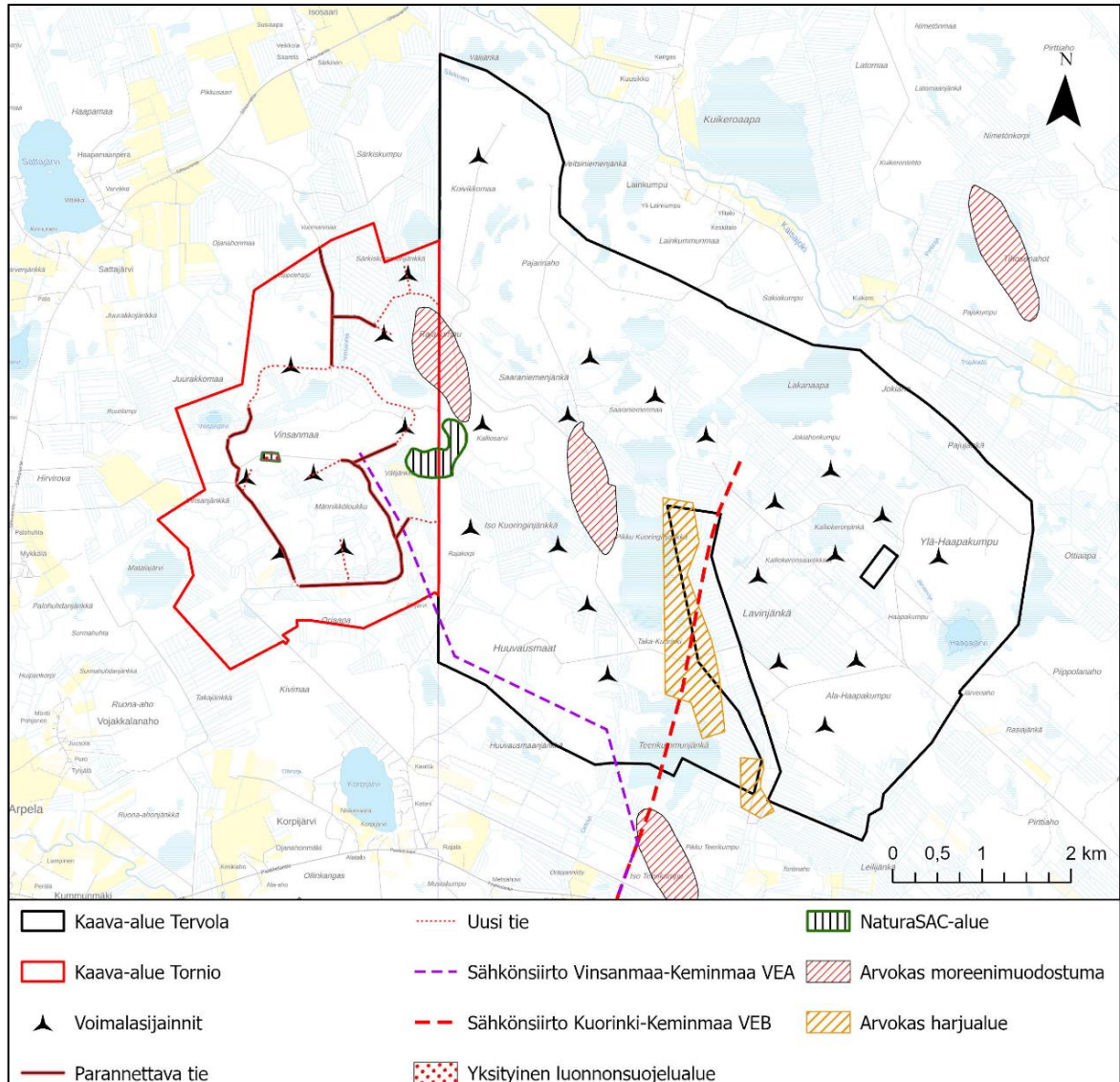
Kuva 4.8. Suojelualueverkoston kohteet suunnittelualueen lähialueilla.
