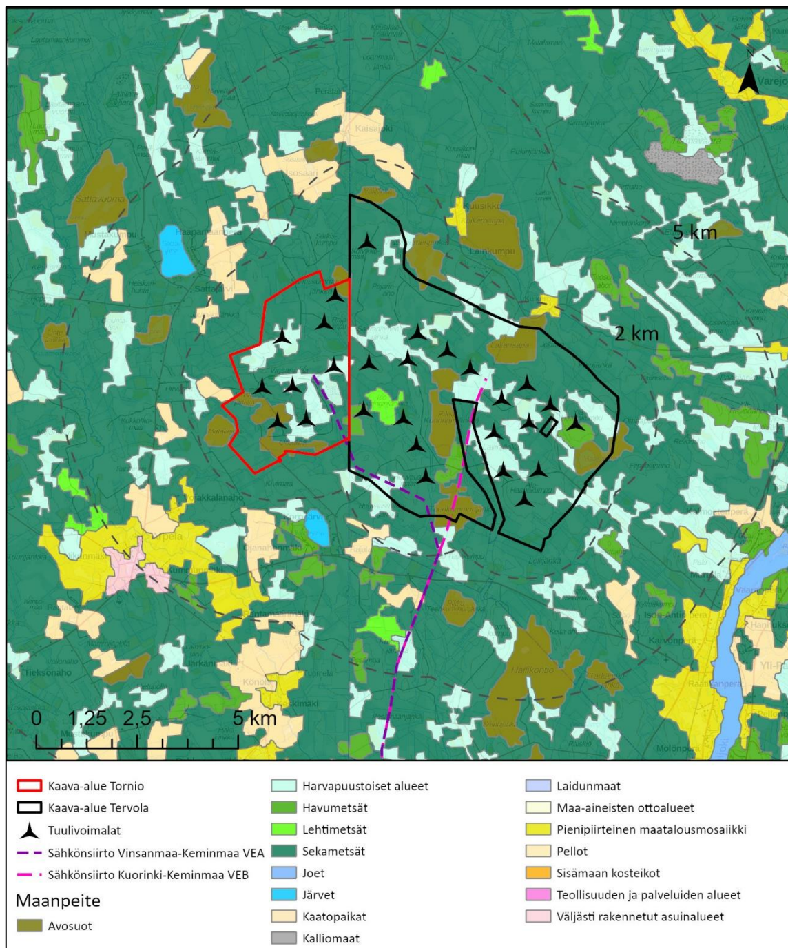
Kuva 4.3. Maanpeite suunnittelualueella ja sen ympäristössä.
