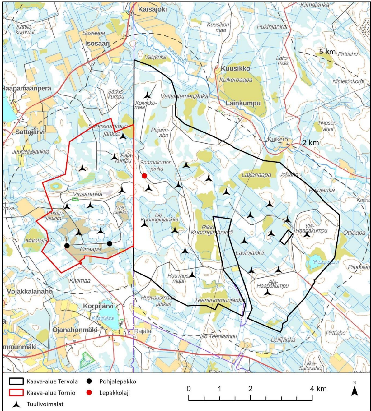
Kuva 4.12. Lepakkoselvityksessä tehty lepakkohavainnot.
