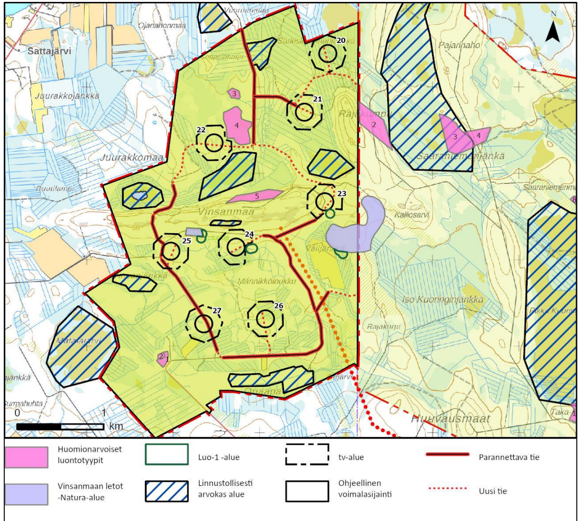
Kuva 4.7. Suunnittelualueella olevat huomionarvoiset luontotyyppikohteet. Kuvaan on merkitty voimaloiden sijainnit ja tiestö.
